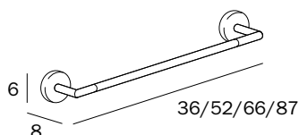
A3618C CR cm 66 x 6H x 8 ●—● cm 60 ● mm 16
