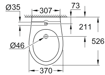
39 433 000 Wall hung bidet
