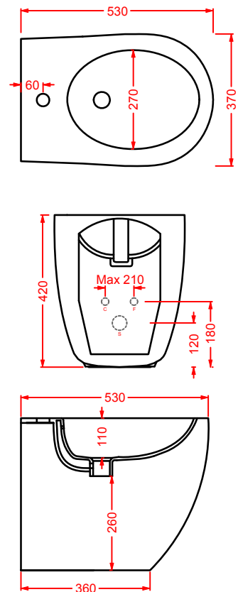
ART ACA034 CURVA TECNICA TRASLATA REGOLABILE DA 15.5 A 21 CM
